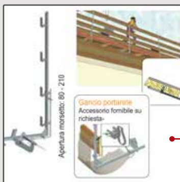
112FR Parapetto frontale per legno
