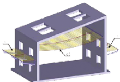
RETE ANTICADUTA
